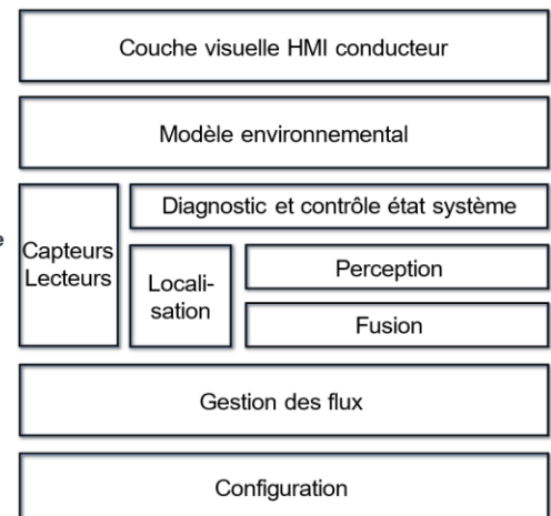
Schéma fonctionnel du logiciel
